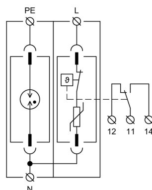
Vnitřní schéma zapojení
